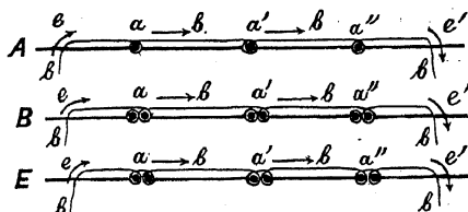
Рис. 78-й. Веденіе нитки при шиваніи на шнурахъ безъ пропилки корешка—швомъ иголкою назадъ . А—шиваніе на оди- ночныхъ шнурахъ; В и Е—шиваніе на двойныхъ шнурахъ.
