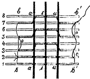
Рис. 75-й. Одинъ способъ шиванія на трехъ шнурахъ по двѣ тетради.
