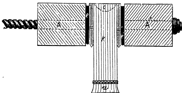
Рис. 109-й. Зажиманіе книги для золоченія передка: A A' — прессъ; к — книга, и — корешокъ, o — передокъ; a и a' — скошенныя по плоскости шпальты; e и e' — нескошенныя (плоскія) шпальты.
