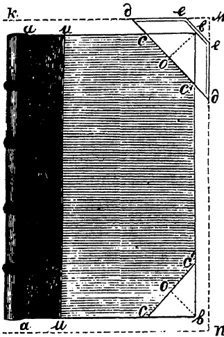
Рис. 130-й. Выкройка кожи для угловъ.
