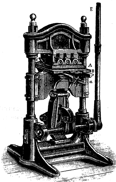
Рис. 169-й. Рычажный прессъ для тисненiя на переплетѣ.
