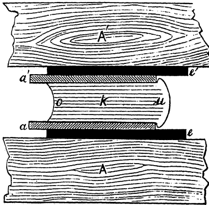
Рис. 110-й. Зажиманіе книги для волоченія головки или хвоста. Буквы имѣютъ то-же значеніе, что на рис. 109-мъ.
