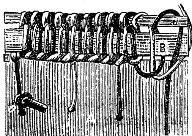
Рис. 122-й. Плетение двойного капитала въ двѣ нитки: u —узенькая полоска картона (или проклеенный шнурокъ и т. п.); значеніе остальныхъ буквъ то-же, что на рис. 118-мъ.
