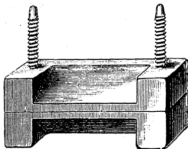
Рис. 32-й. Тиски для золоченія.
