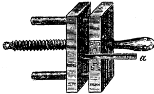
Рис. 6-й. Гобель; a —рѣзакъ.
