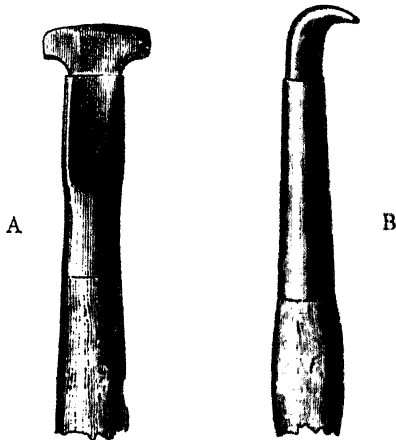
Рис. 108-й. А—плоскій лохильный зубъ; В—закругленный и заостренный лохильный зубъ ( волчий зубъ ).
