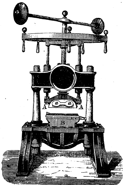
Рис. 168-й. Винтовой прессъ для тисненія на переплетѣ.
