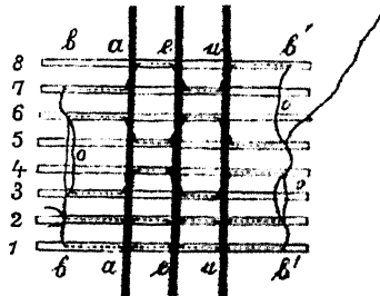
Рис. 76-й. Другой способъ шиванія на трехъ шнурахъ по двѣ тетради.
