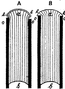
Рис. 82-й. Книга, зажатая въ прессъ между дощечками o и o ; α —корешокъ, o —обрѣзъ передка; e и e —фальцы. А—до сколачиванія фальцовъ, В—послѣ околачиванія фальцовъ на корешкѣ.
