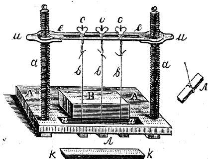
Рис. 1-й. Швальный станокъ.
